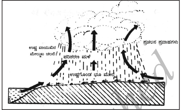
ಪರಿಸರಣ ಮಳೆ
