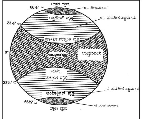
ಉಷ್ಣಾಂಶ ವಲಯಗಳು
