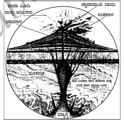
ಜ್ವಾಲಾಮುಖಿ ರಚನೆ
