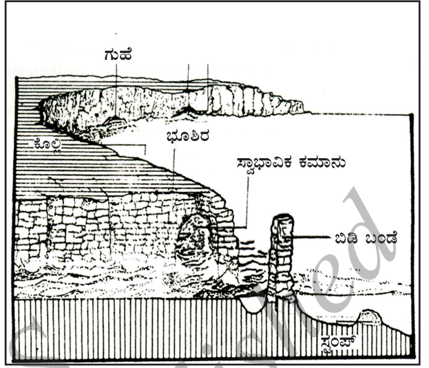
ಸಮುದ್ರದ ಅಲೆಗಳು
